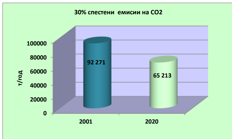
Фиг. 5.11. Въздействие на всички мерки и очаквани резултати за намаляване на емисиите на CO 2 в община Карлово през 2020 г.
