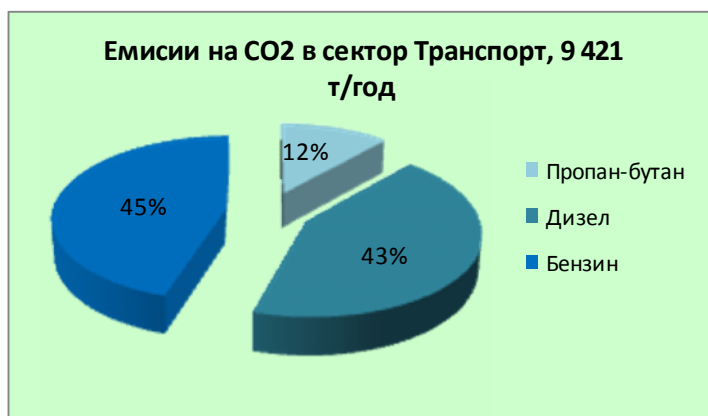
Фиг. 2.8. Структура на емисиите CO 2 от горива в сектор „Транспорт”
